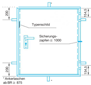
Feuerschutzwandklappe: Ansicht, Horizontalschnitt
