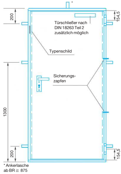
Feuerschutztür: Ansicht, Horizontalschnitt
