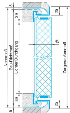
Feuerschutzwandklappe: Vertikalschnitt
