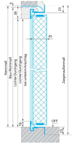
Feuerschutztür: Vertikalschnitt
